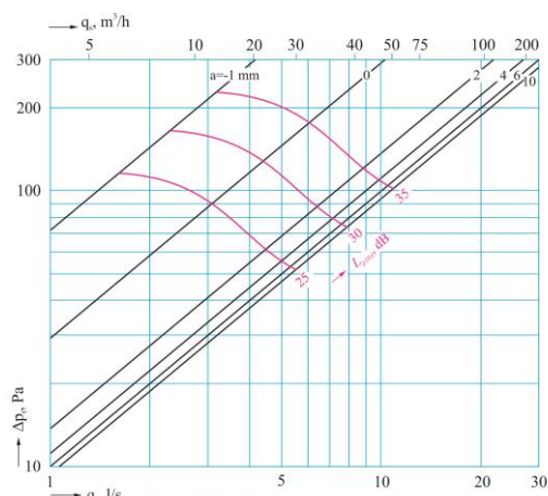
DVSC-P 080 mm
