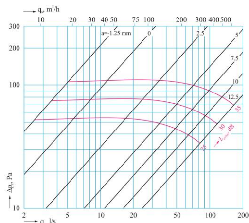
DVSC-P 200 mm
