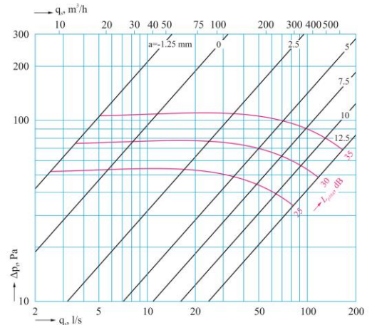
DVS-PY 200 mm
